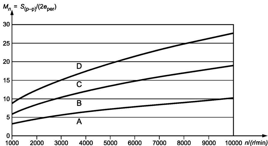
Рисунок 3 — Границы зон вибрационного состояния согласно [2] и [3]
