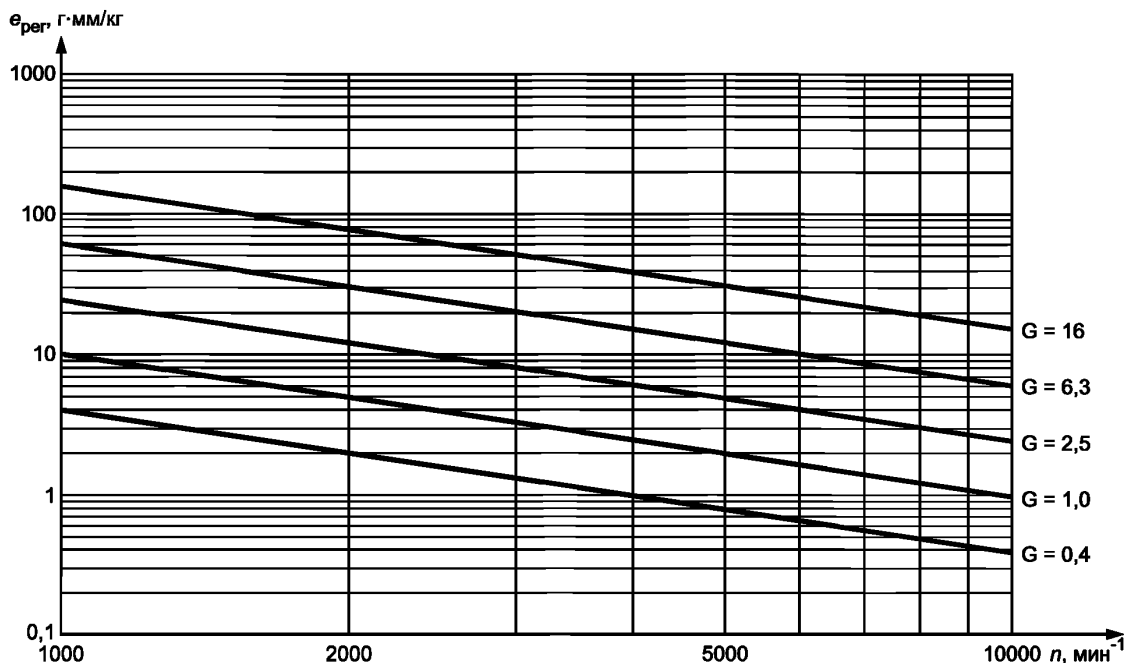
Рисунок 1 — Допустимый удельный дисбаланс по [1]
