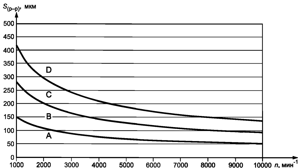
Рисунок 2 — Границы зон вибрационного состояния согласно [2] и [3]
