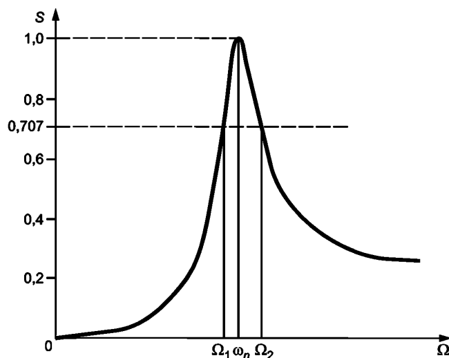
Рисунок 6 — Применение диаграммы Бодэ для оценки модальной чувствительности
